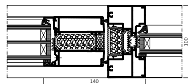
Section latérale de la porte et de la fenêtre fixe
