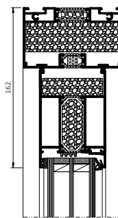
Section de la partie supérieure de la porte
