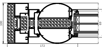
Partie latérale de la porte avec serrure de sécurité
