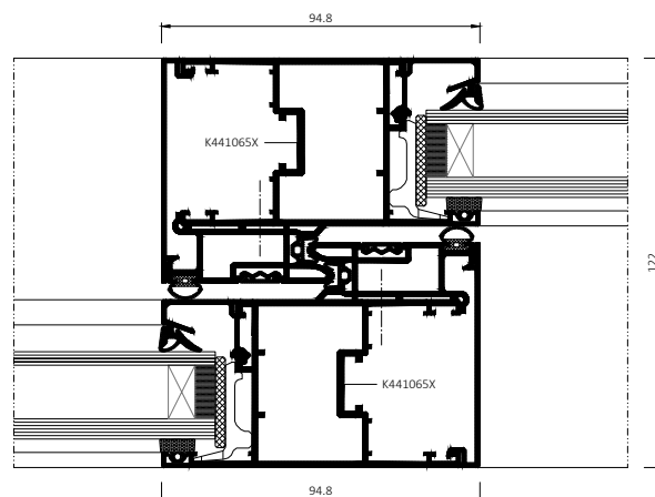
Przekrój przez połączenie skrzydeł drzwi
