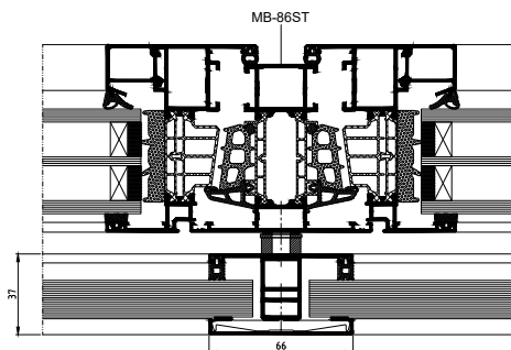
Schnitt durch den Fensterpfosten mit Brüstungsverglasung
