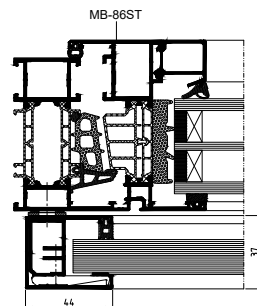
Fenster mit Brüstungsverglasung Schnitt
