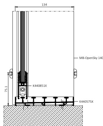
Panneau et seuil MB-Open Slide
