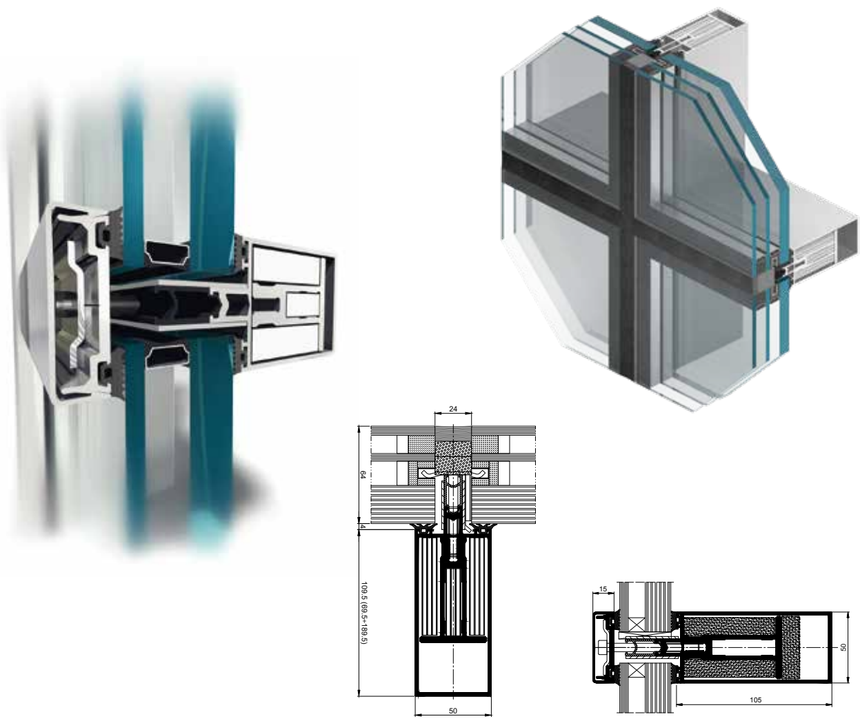
mullion – cross-section EI 45, EI 60
