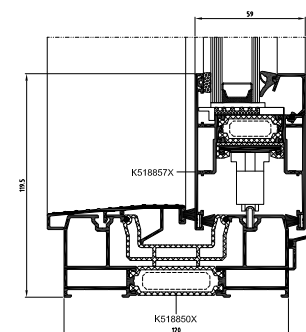
przekrój dolny drzwi
