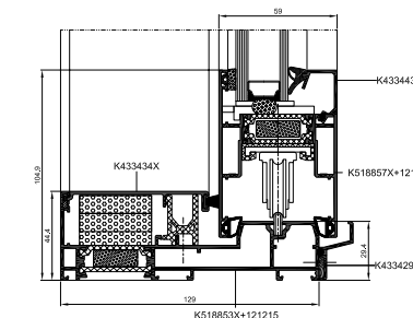
przekrój dolny drzwi z oknem stałym
