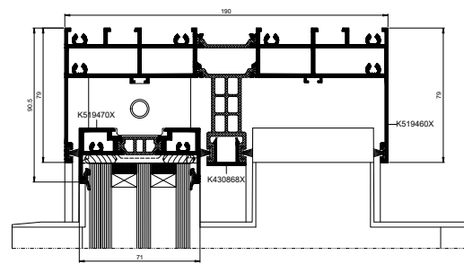
przekrój górny drzwi
