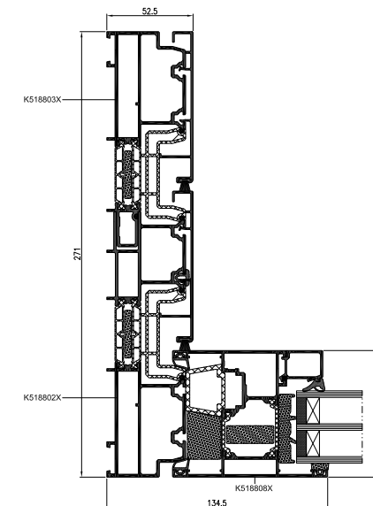
przekrój przez drzwi z ościeżnicą 3-szynową
