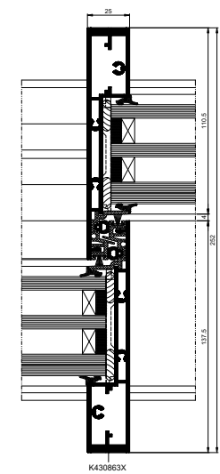
przekrój przez połączenie skrzydeł drzwi
