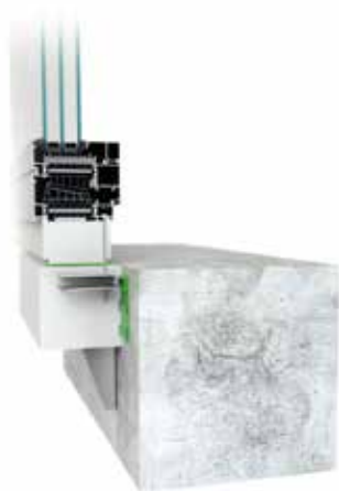
połączenie dolne, na belce 100 mm z kotwą zewnętrzną
