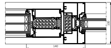
Przekrój boczny przez drzwi (SI) i okno stałe
