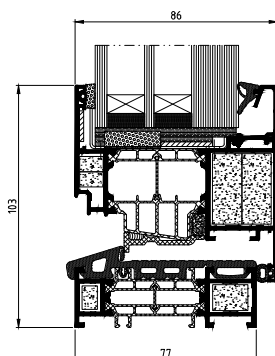
przekrój przez drzwi z niskim progim
