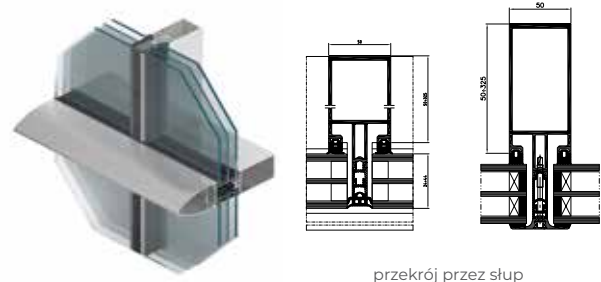
przekrój przez słup
