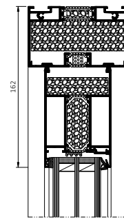
Przekrój górny drzwi (SI)
