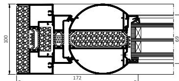
Przekrój przez bok drzwi (SI) z bezpiecznym przymykkiem
