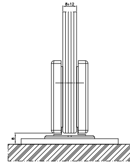
przekrój dolny drzwi
