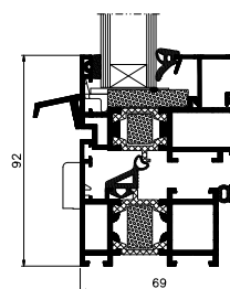
przekrój okna
