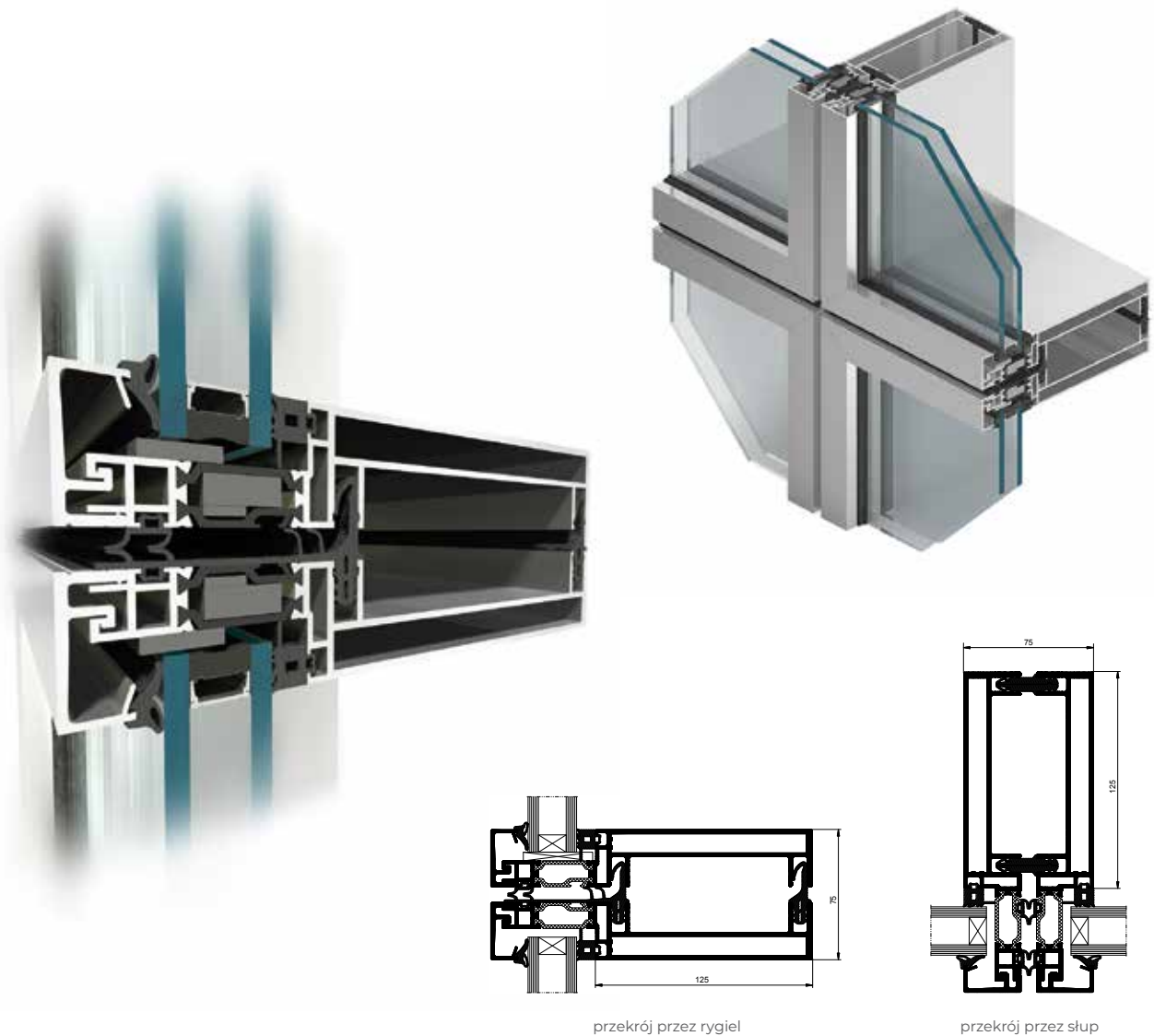
przekrój przez rygiel
