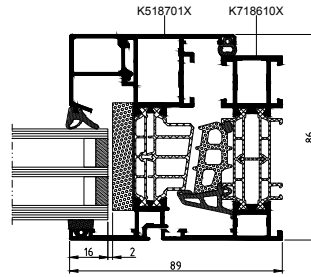
doorsnede raam
