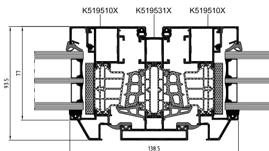
Сечение по стойке и открываемым окнам
