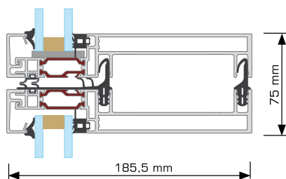
Riegel - Schnitt
