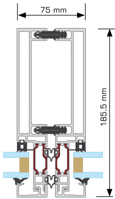
Pfosten - Schnitt
