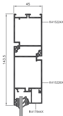
Querschnitt durch den Rahmen und Türflügel
