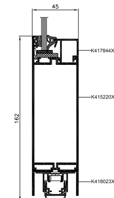
Unterer Querschnitt durch Tür ohne Schwelle
