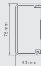
Führungsschienenquerschnitt
