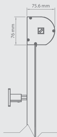
Kassettenabmessungen
