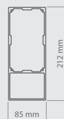
Profilquerschnitt
