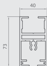
Querschnitt oberes Rahmenprofil
