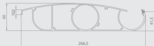
Pfostenquerschnitt
