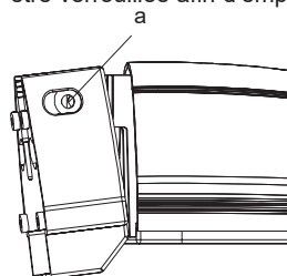
Support mural pivoté à 90°
