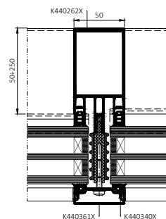
Řez sloupem MB-MT50N SI
