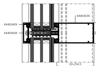
Řez příčkou MB-MT50N SI
