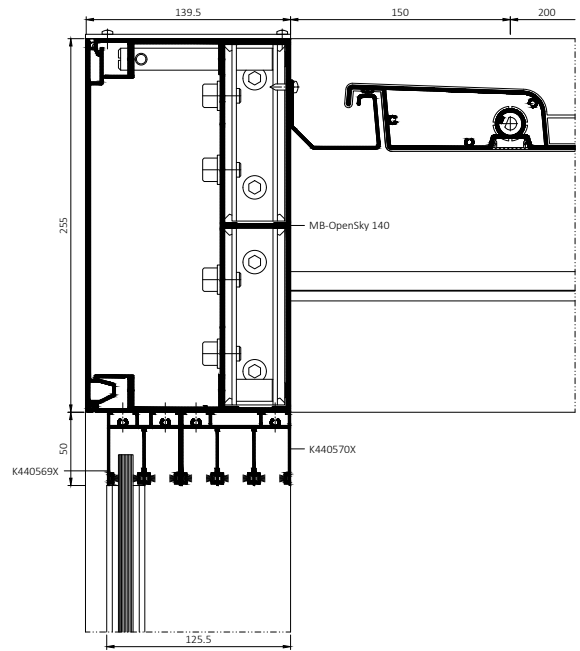
Pergolan yläparrun ja MB-OpenSlide-kehysten poikkileikkaus
