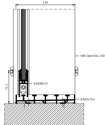
MB-OpenSlide-paneelin ja kynnyksen poikkileikkaus
