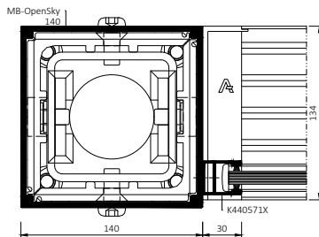
Pergolan pylvään ja MB-OpenSlide-paneelin poikkileikkaus
