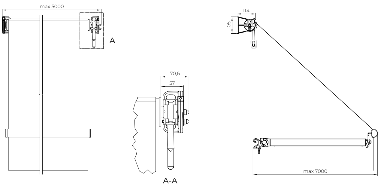
MARKIZA ITALIA PORĘCZOWA Wysięg maksymalny
