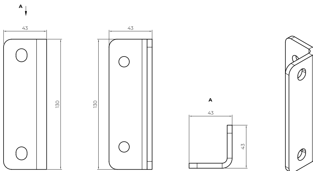
MARKIZA ITALIA Wspornik wewnętrzny
