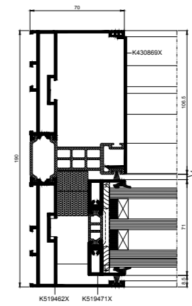
Seitlicher Schnitt der Tür
