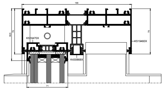
Schnitt Türoberseite
