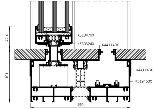
Schnitt Türunterseite
